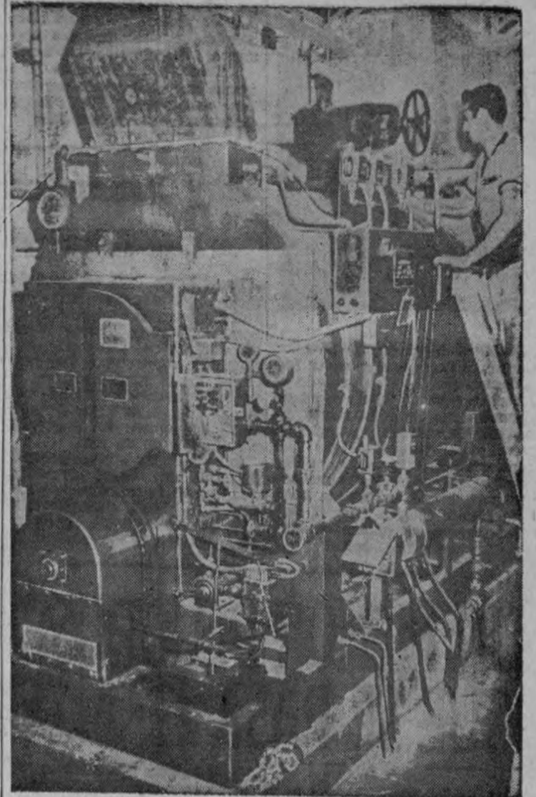
LA NUEVA CALDERA.—Esta enorme caldera, que desplaza 100 caballos de fuerza, fue importada en 1958 para sustituir a una de 30 caballos que ahora opera en el Hospital de Turrialba. El resultado que se ha obtenido con este nuevo tipo de caldera ha sido magnífico, mejorando en mucho el servicio de la lavandería y bajando los costos de operación
