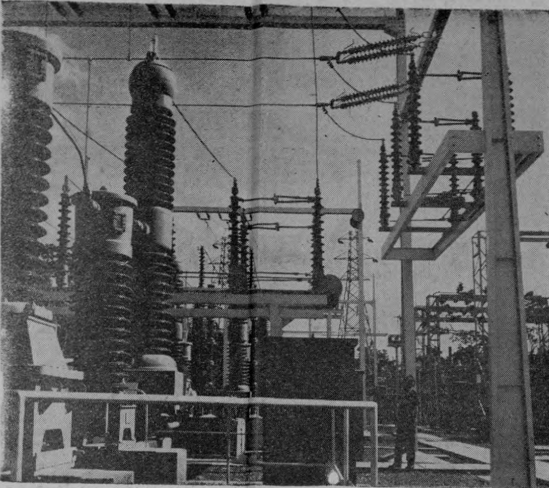
Vista de una de las Sub-Estaciones del ICE. Obras modernas y eficientes.
