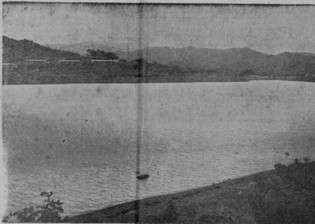
Embalse de la Planta Hidroeléctrica de La Garita funcionando para regular el caudal del Río Grande. La Garita genera en la actualidad 34.000 KW de máxima demanda y produce mensualmente 13.000.000 de KW/H. En la estación seca La Garita opera sin faltante de agua y su producción es mayor que la de todas las otras plantas hidroeléctricas juntas.
